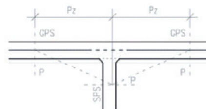
Slika 2a: Priključevanje brez priključnih zavijalnih lokov
